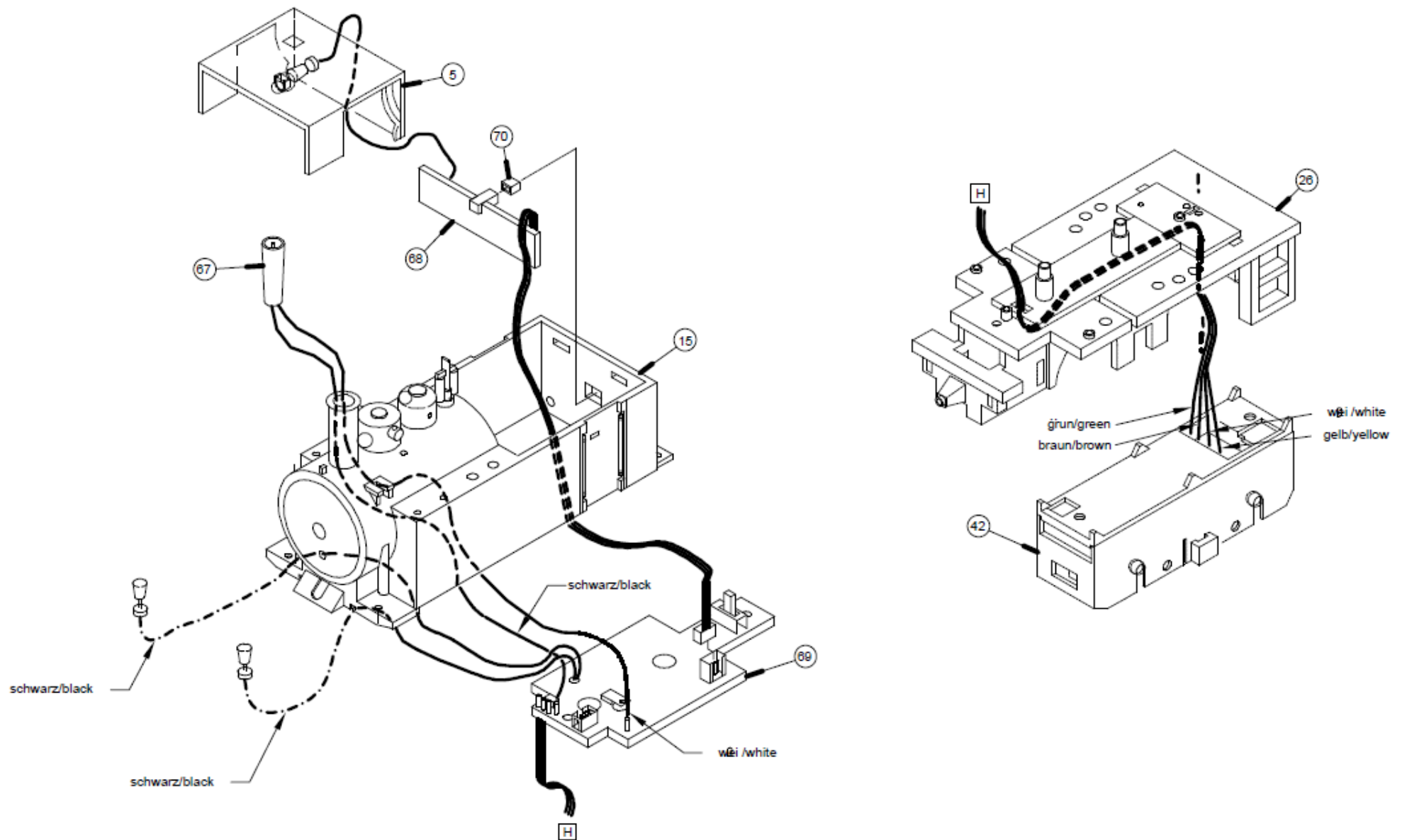
Einzelteile der Lokomotive 20761
