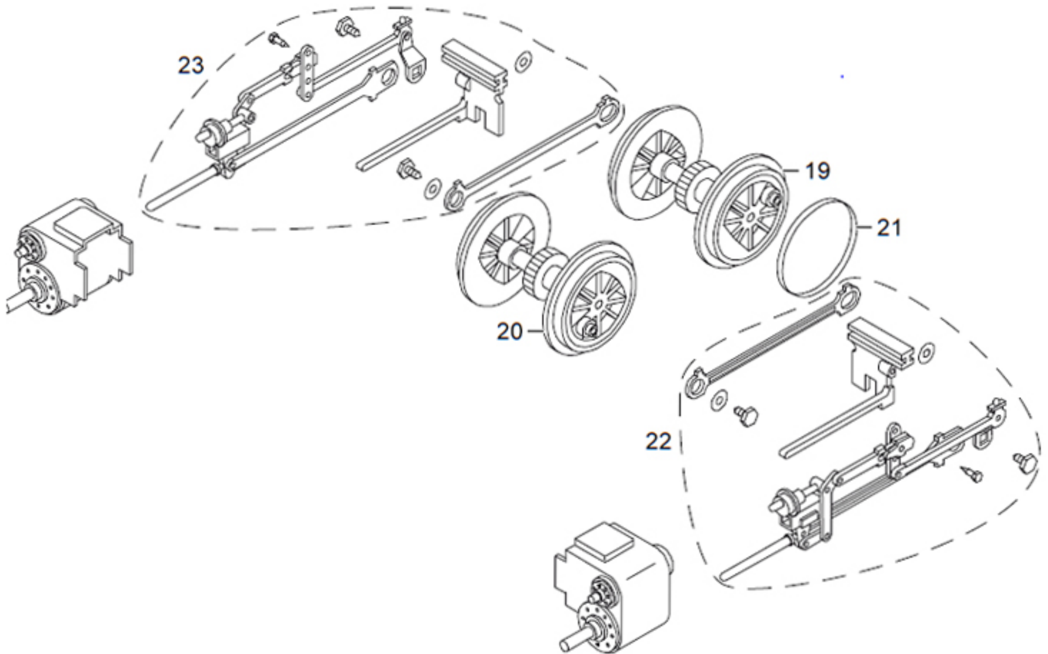
Einzelteile der Lokomotive 20752
