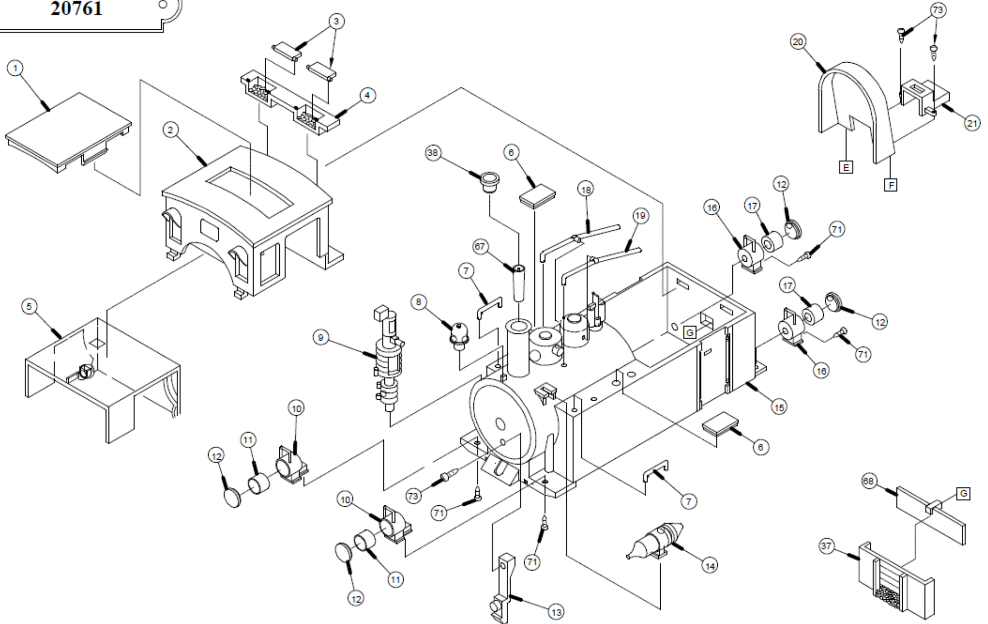
Einzelteile der Lokomotive 20761
