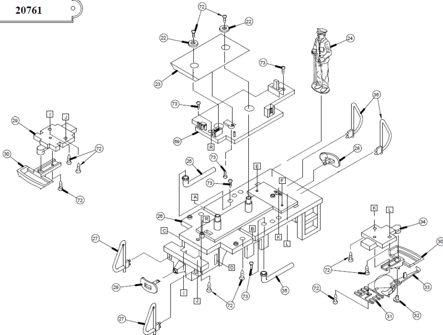
Einzelteile der Lokomotive 20761
